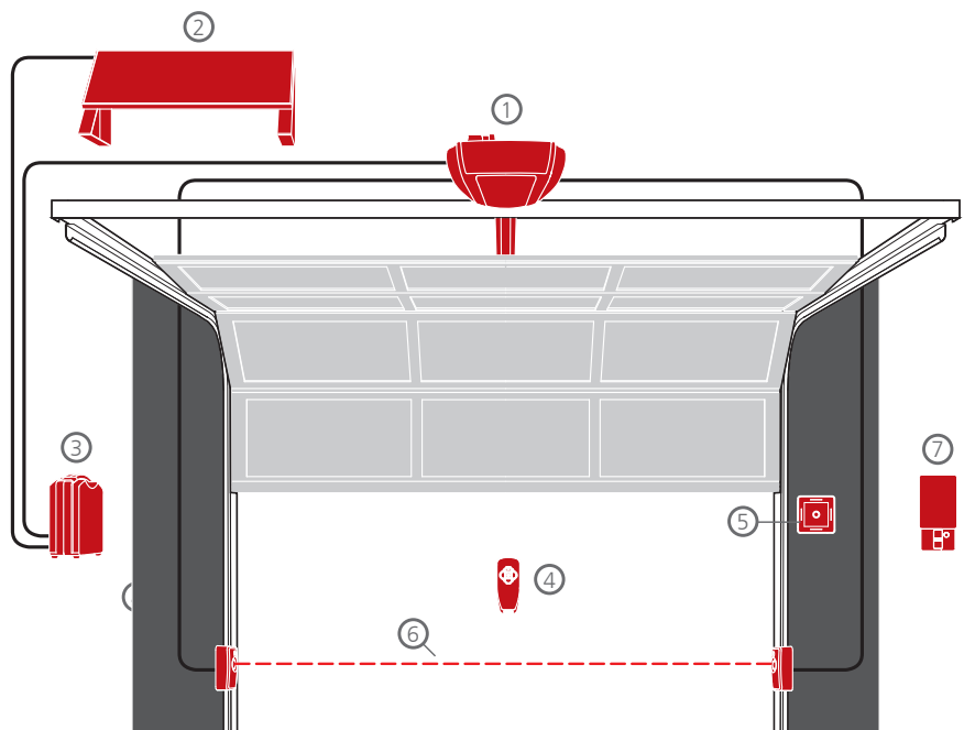
Unsere Antriebsschienen sind absolut wartungsfrei und durch ihr hochwertiges Zahnriemensystem extrem leise.
